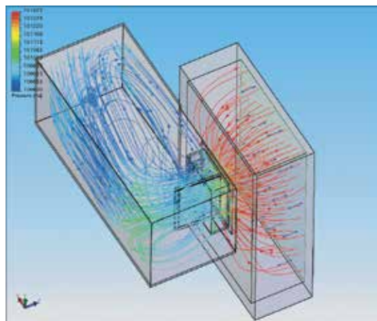
Линии тока с распределением давлений в «стенном» клапане КЛАД®-2
