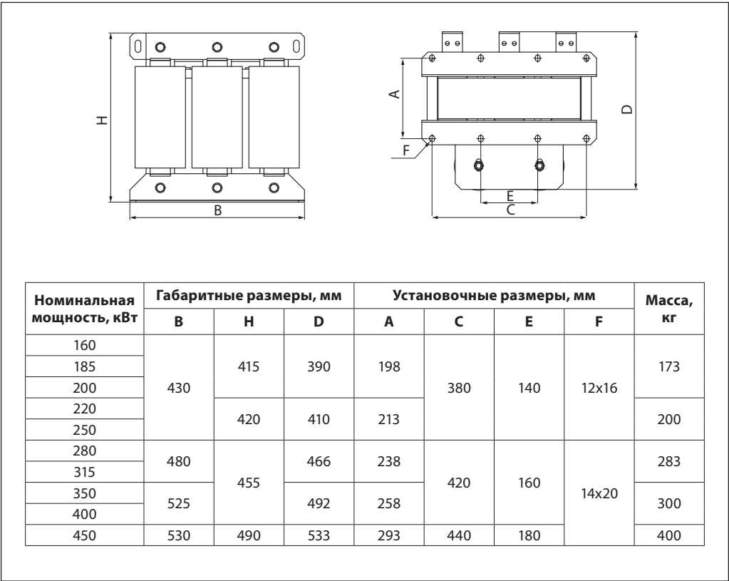
Синус-фильтр типоразмер 3
