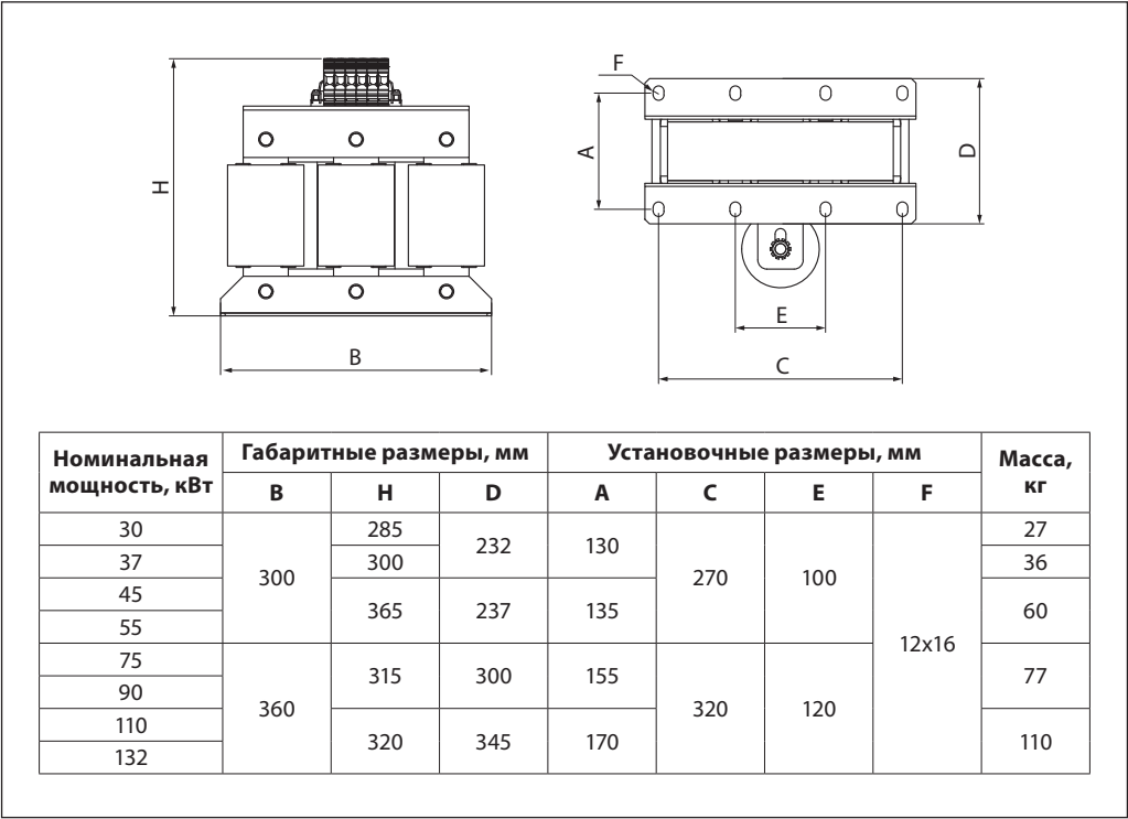
Синус-фильтр типоразмер 2
