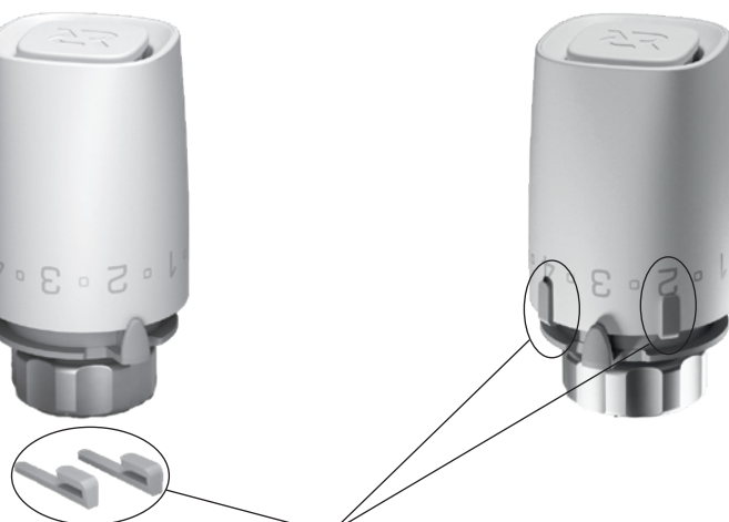
Фиксаторы настройки (входят в комплект поставки)
