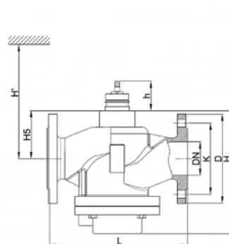
Клапан AQF-R DN 65-200
