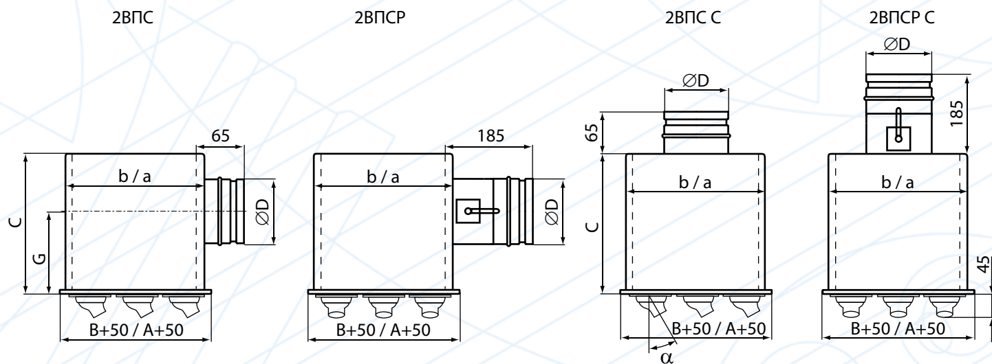
Конструктивные схемы воздухораспределителей 2ВПС, 2ВПСР
