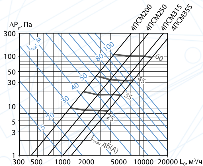
Аэродинамические и акустические характеристики 4PCM при подаче воздуха в помещение прямооточными струями вдоль оси сопла
