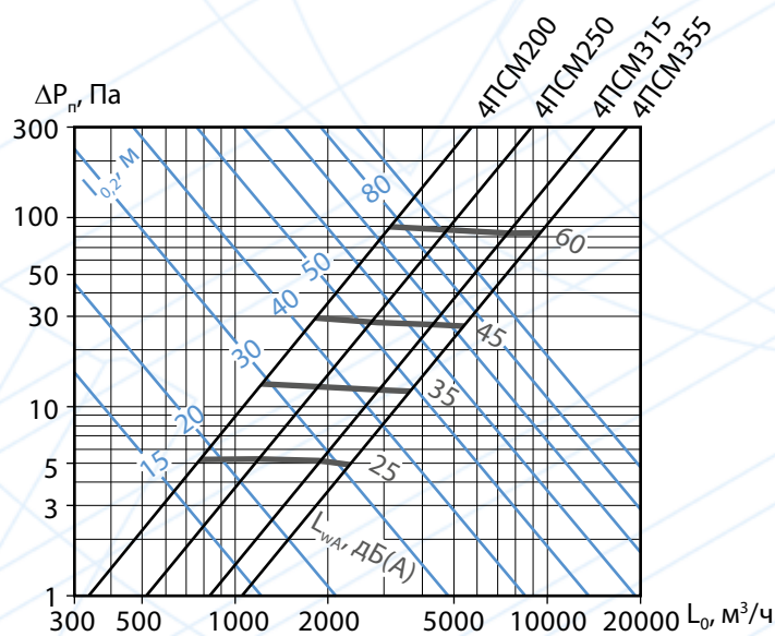
Аэродинамические и акустические характеристики 4PCM при подаче воздуха в помещение наклонными струями под углом 25° к оси сопла
