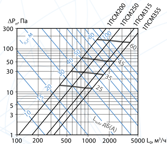
Аэродинамические и акустические характеристики 1PCM при подаче воздуха в помещение прямооточными струями вдоль оси сопла
