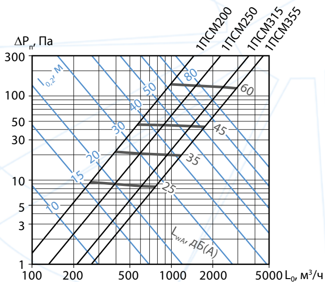
Аэродинамические и акустические характеристики 1PCM при подаче воздуха в помещение наклонными струями под углом 30^\circ к оси сопла
