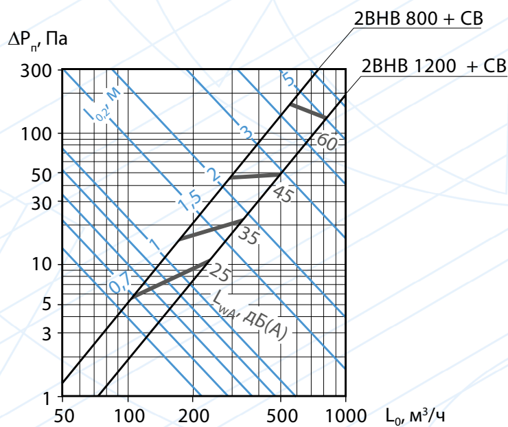
Аэродинамические и акустические характеристики воздухораспределителей 2BHB 800 + CB, 2BHB 1200 + CB при подаче воздуха в помещение
