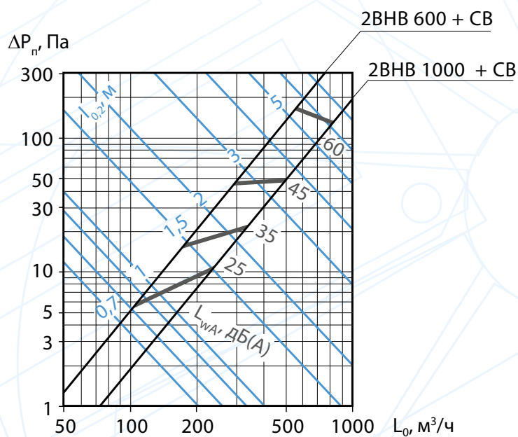
Аэродинамические и акустические характеристики воздухораспределителей 2BHB 600 + CB, 2BHB 1000 + CB при подаче воздуха в помещение
