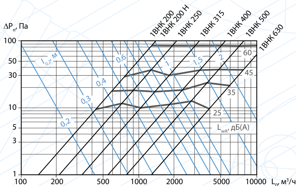
Аэродинамические и акустические характеристики воздухораспределителей 1ВНК при подаче воздуха в помещение
