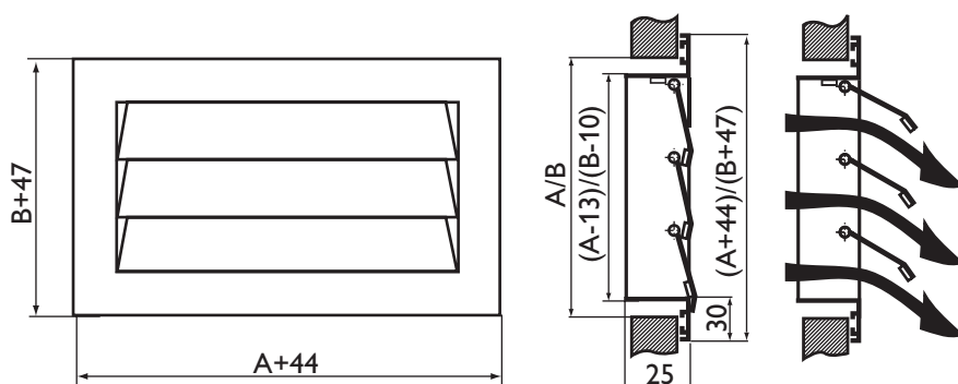
Данные для подбора инерционных решеток АГС
