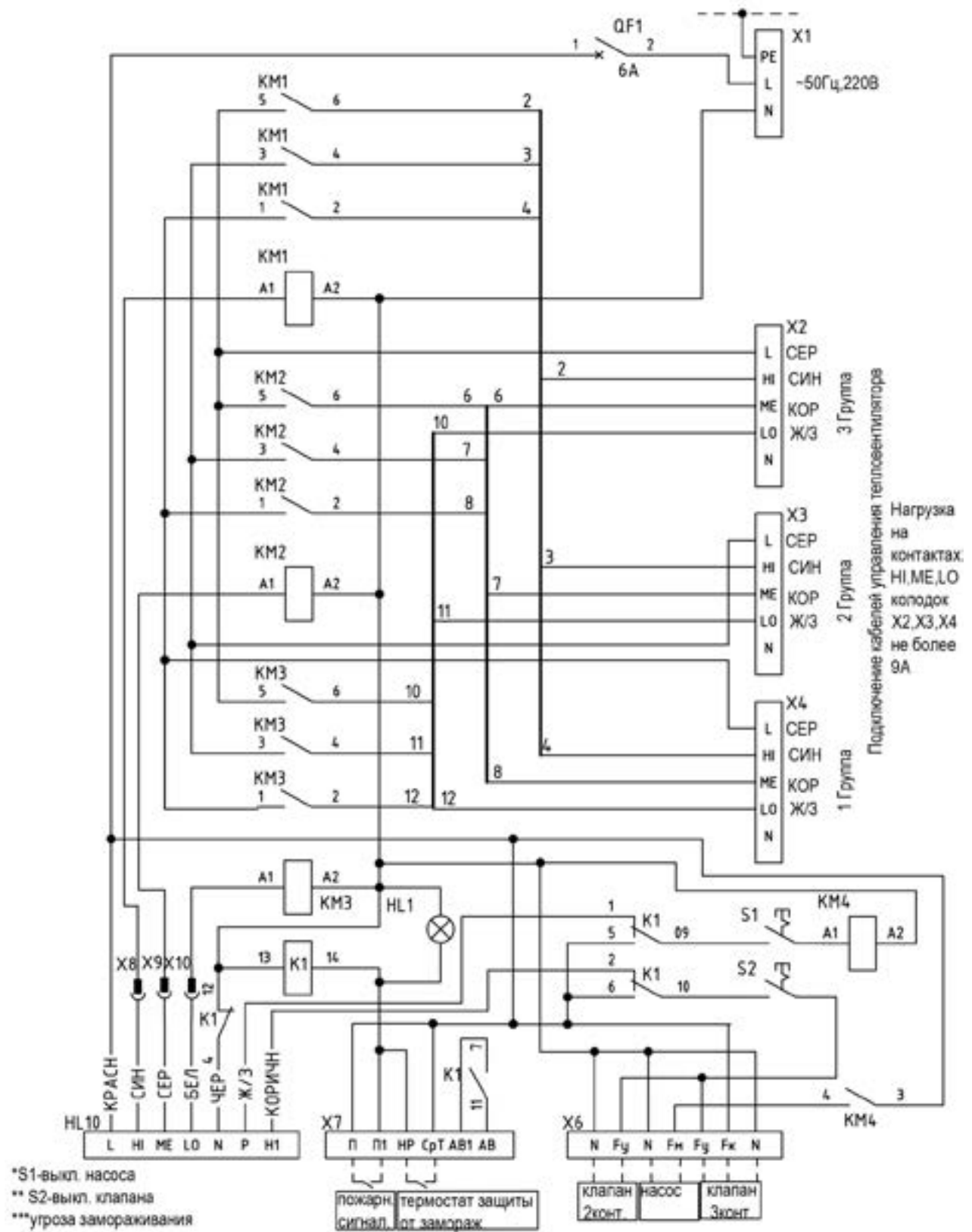
Электрическая схема пульта коммутации и управления ПКУ-W1
