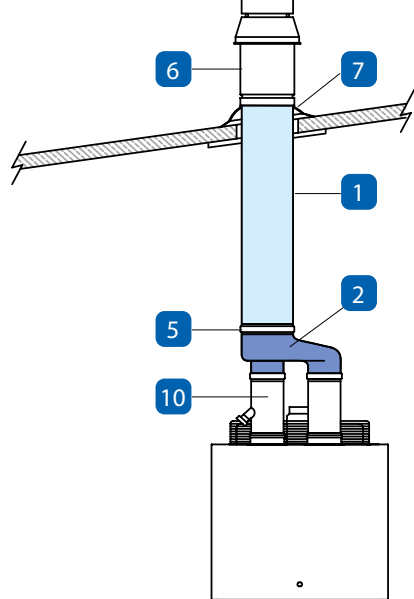
Для воздухонагревателей серии 45/55/75/95TV
