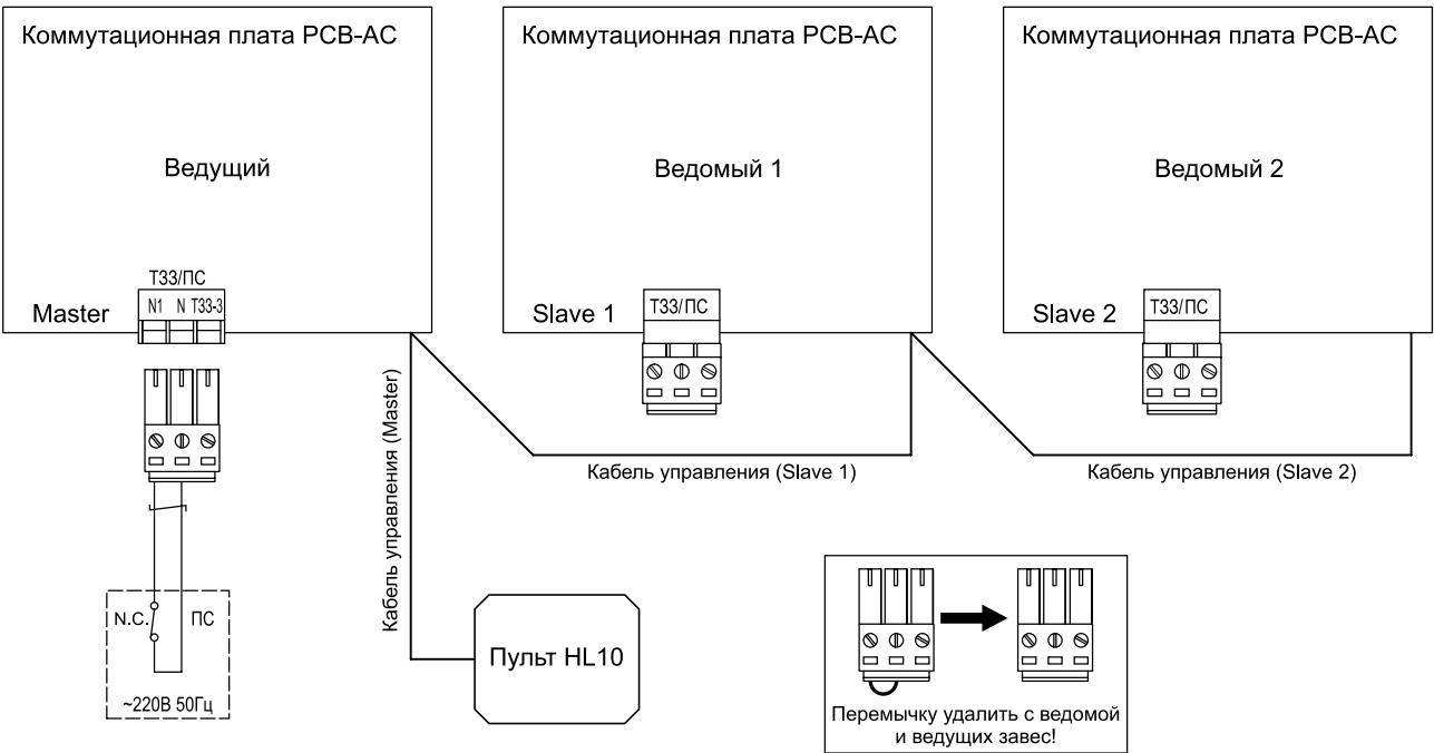
СХЕМА ПОДКЛЮЧЕНИЯ ПС К ГРУППЕ ЗАВЕС БЕЗ ИСТОЧНИКА ТЕПЛА
