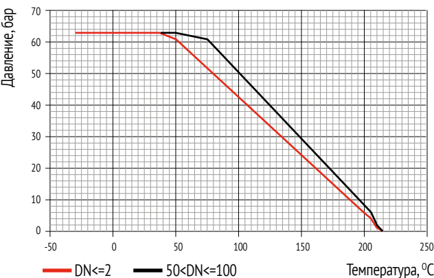
Диаграмма температура/давление
