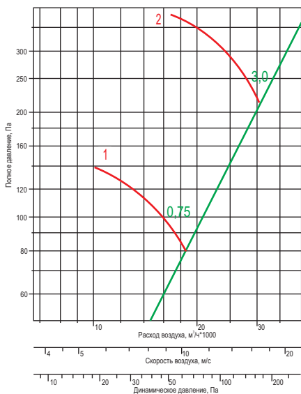
ВО 12-303-8-В
