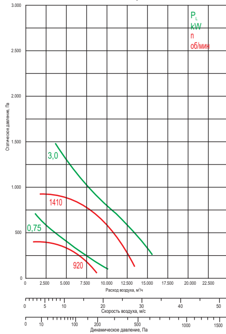
BP 80-75-5,6-B-...
