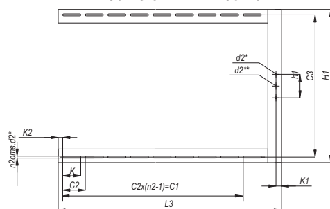
ВР 80-75-9 - ВР 80-75-11
