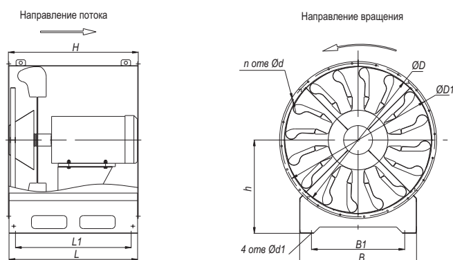
Компоновка 02
