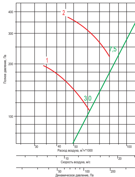
ВО 12-303-12,5-В
