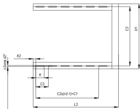
ВР 80-75-9 - ВР 80-75-11
