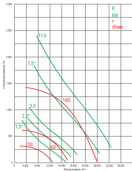
ВКР-7,1-В-С-...
