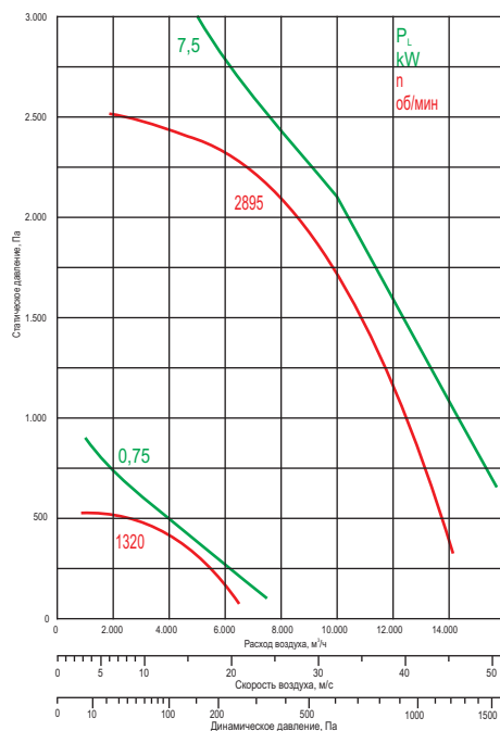
BP 80-75-5,6-B-...
