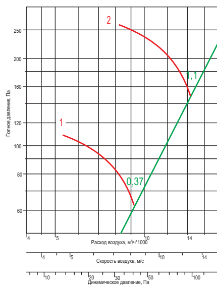
ВО 12-303-6,3-В
