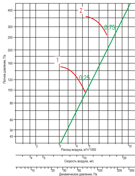
ВО 12-303-4-В
