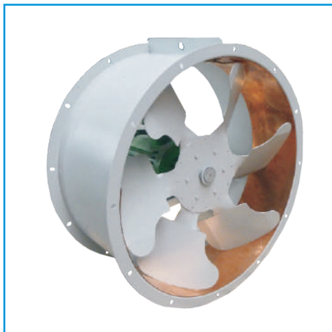
Вентилятор осевой типа ВО 25-188-B
